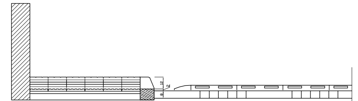
SECCIÓ B - B'
