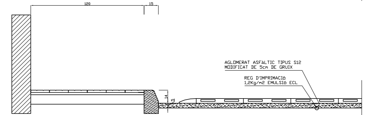
SECCIÓ C - C'
