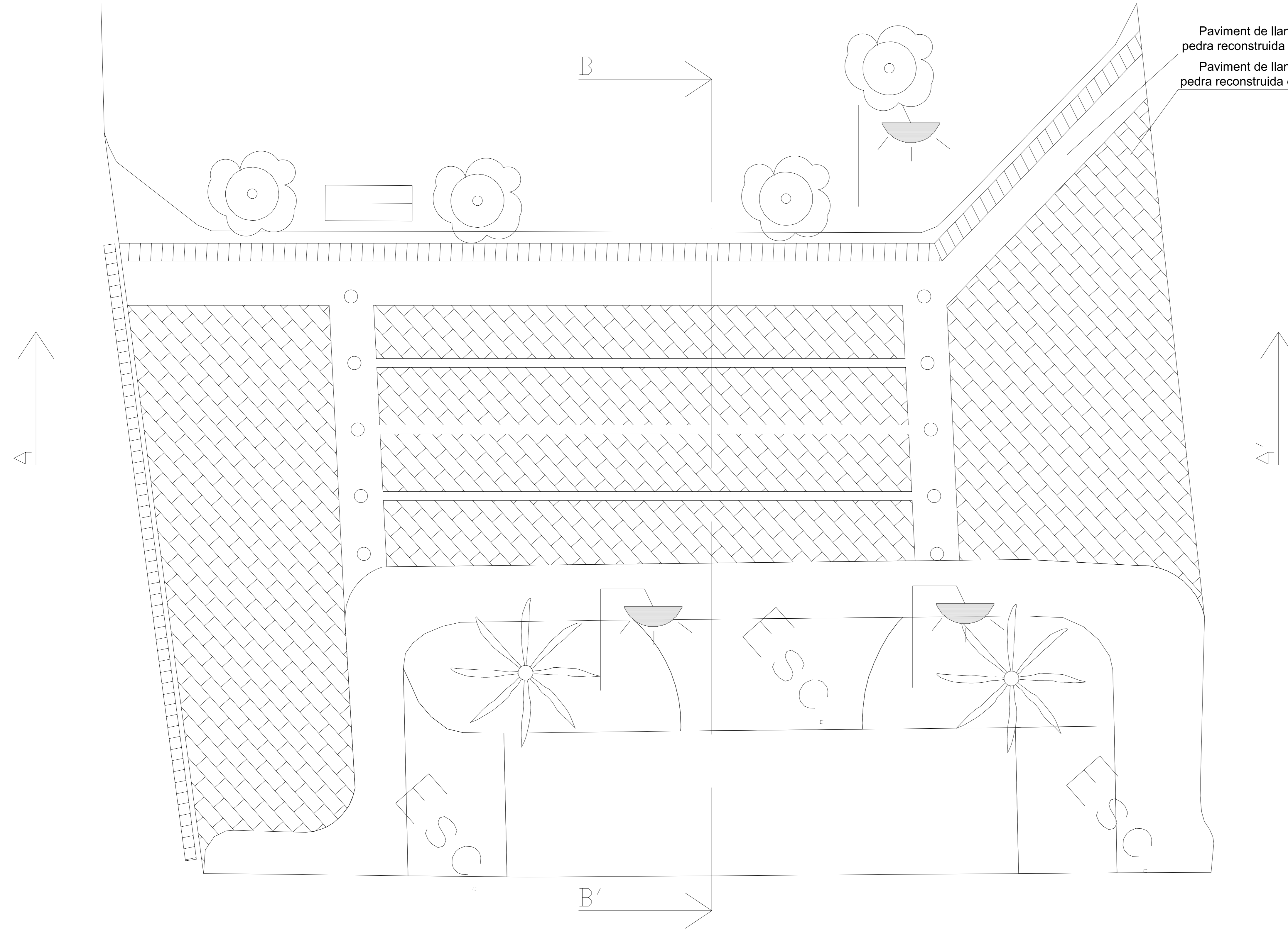
PLANTA
