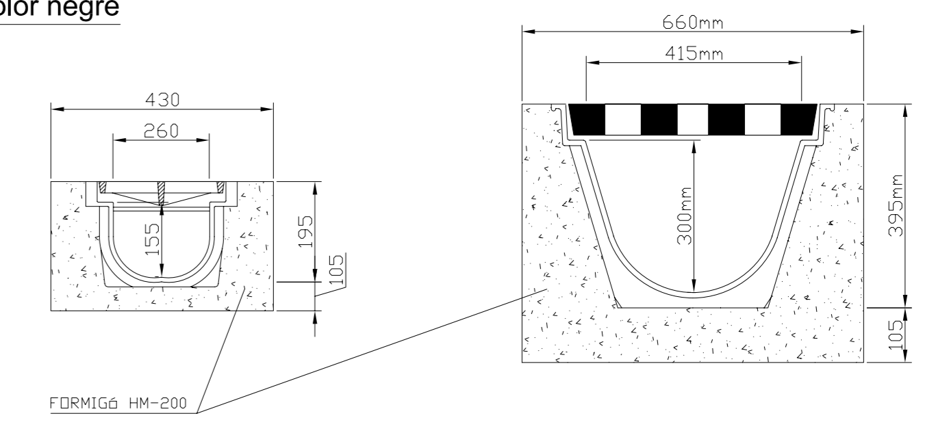
DETALL CANALETES
