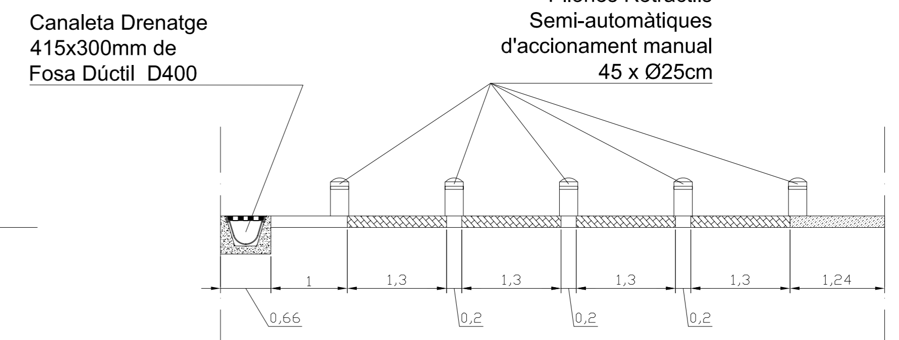
SECCIÓ B-B'
